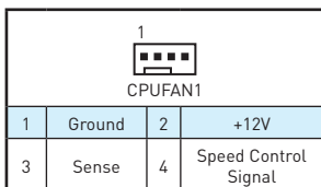
PWMモードファンコネクタ
