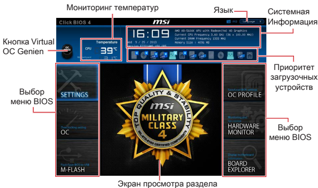
Экран просмотра раздела
