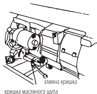
кришка масляного щупа
