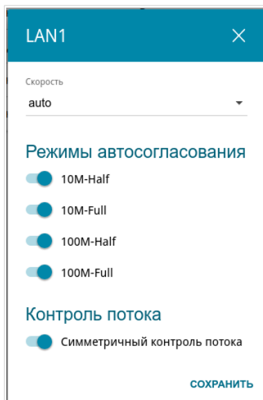
Рисунок 96. Окно изменения настроек порта маршрутизатора.
