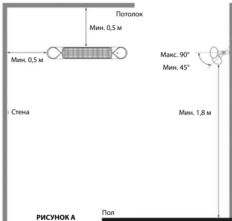
Рисунок 2: Правильная установка на стене/потолке
