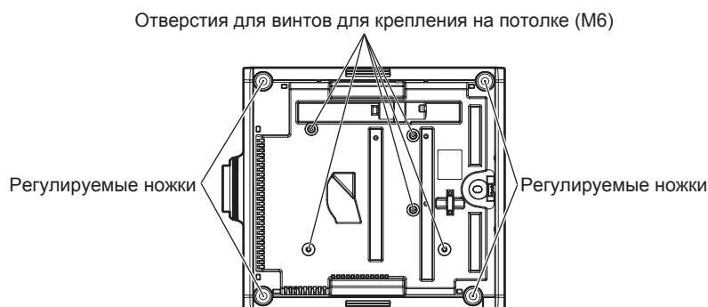
Положения отверстий для винтов для крепления на потолке и регулируемых ножек
