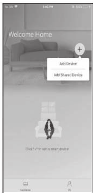
Android
