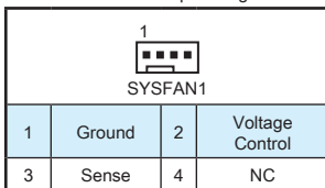
Lüfteranschluss des Spannungs-Modus
