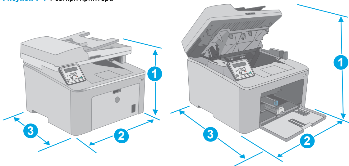
Рисунок 1-1 Розміри принтера
