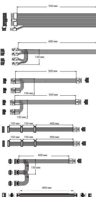
Разъемы питания материнской платы
