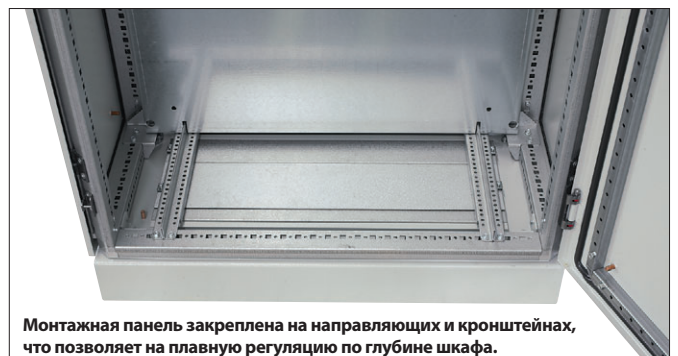
Направляющие монтажной панели
