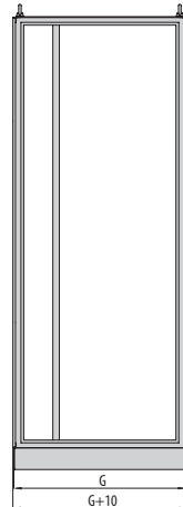
Вид с боку (шкаф без боковых стенок)
