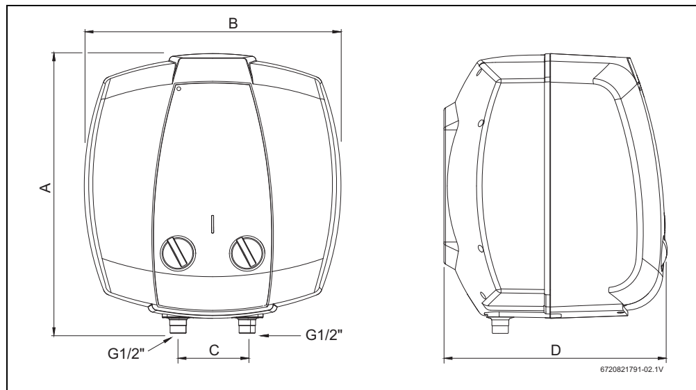
Мал. 2 Розміри в мм
