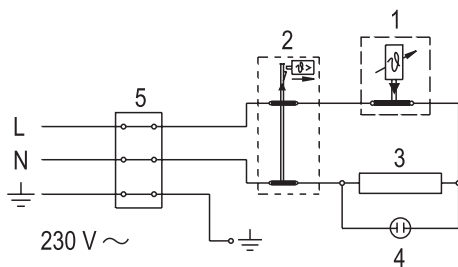
Схемa на електрично поврзување
