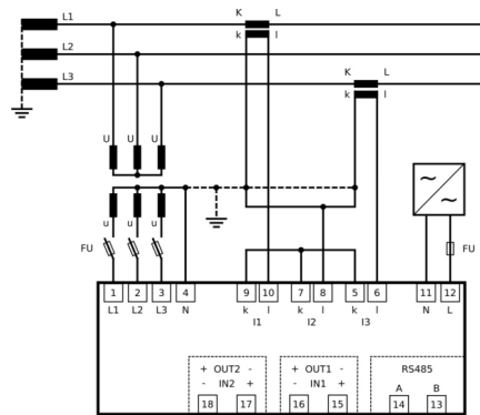
Подключение сети среднего напряжения
