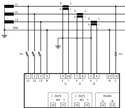
Измерение в трехфазной сети
