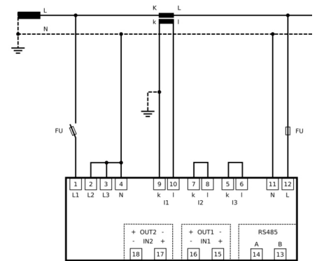
Измерение в однофазной сети
