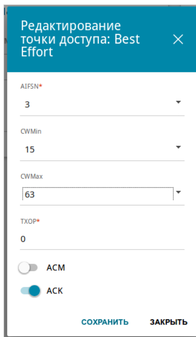
Рисунок 103. Окно для изменения параметров функции WMM.
